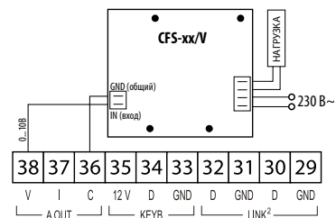
FH аналоговый выход 0...10 В с внешним модулем CFS-xx/V
